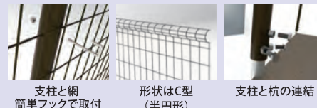
部品写真及び取付け用具
